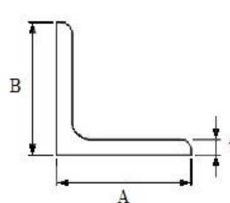
山形鋼
