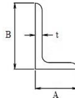
不等辺山形鋼
