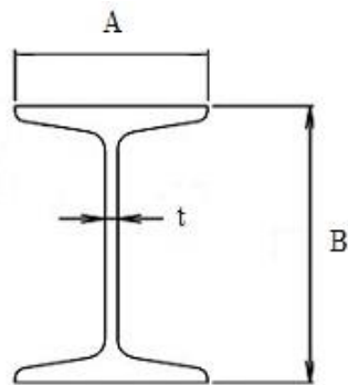
I形鋼
